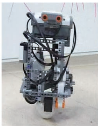
卒業研究：ボールバランスロボット Graduation Research: Ball Balance Robot
