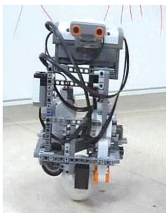
卒業研究：ボールバランスロボット
